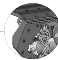
Châssis très robuste avec plaques d'usure interchangeables pour une très longue durée de vie du broyeur
