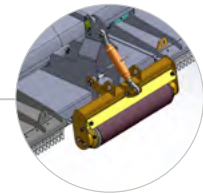
Selon les exigences, avec rouleau (standard) ou roues arrière pivotante (option)
