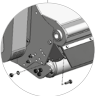
Capó regulable para regular el grado de trituración del producto M-FLAP
