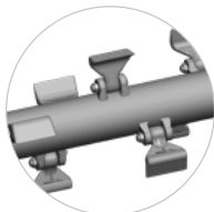
Rotor estándar con martillos SMW
