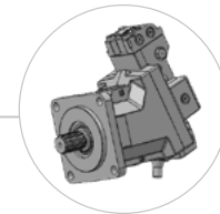
Motor M-BOOST (1-2) mit automatischer Schluckvolumenregelung und Überdruckventil
