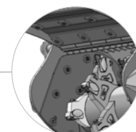
Austauschbare Verschleißplatten im Gehäuse und unter der Haube für eine lange Lebensdauer
